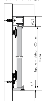
Izračun dimenzija ispune
