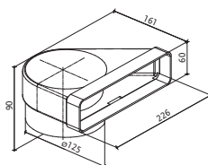
KOLJENO CRV 90 REVERZIBILNO FUN 112.0157.298
