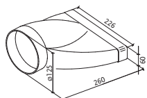
KOLJENO CRV 90 REVERZIBILNO FUN 112.0157.298
